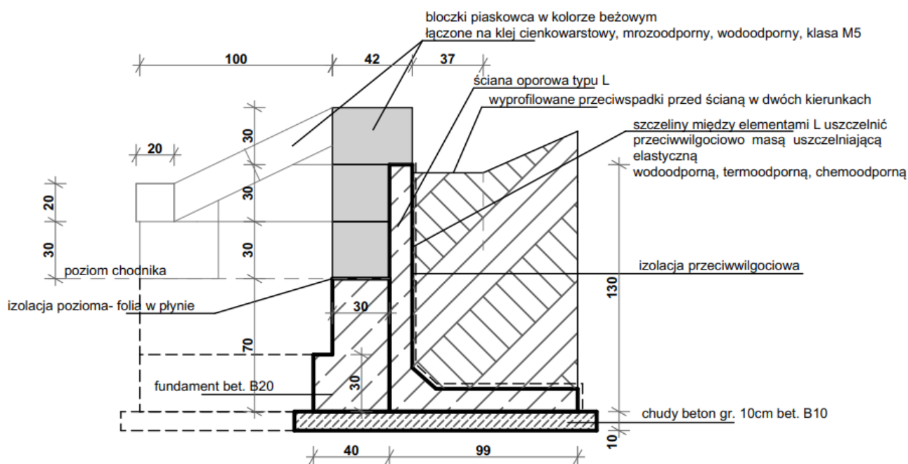
RYСУNEK USZCZEGÓLAWIAJĄCY DO RYSUNKU PAB- 2.1
